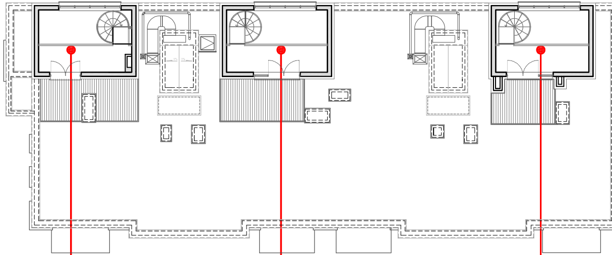
Mieszkanie nr 9 3P+AK+Antresola 77,90 m 2
